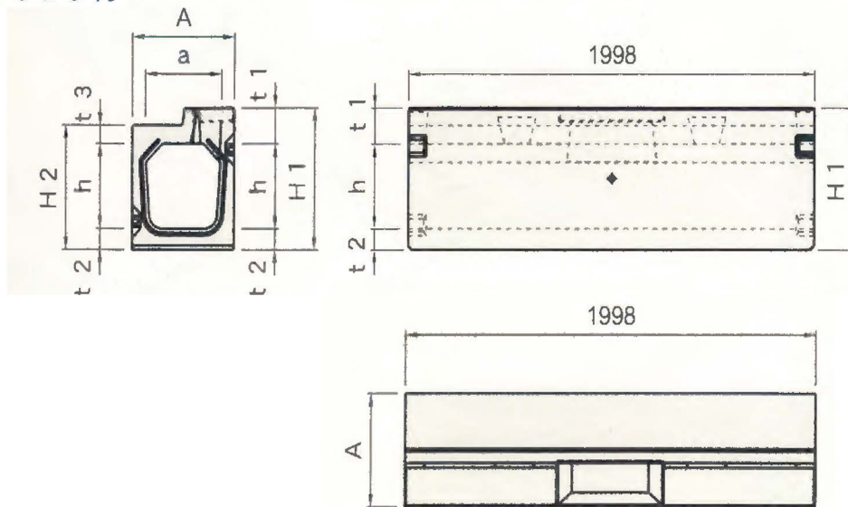
タイプ1 寸法表
