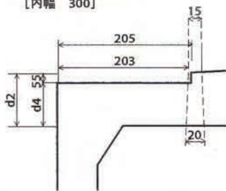
本体上部詳細図
