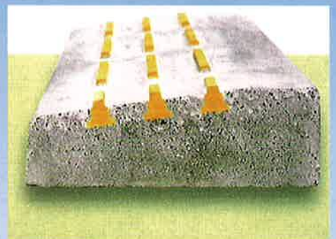
セーフティブロック断面
