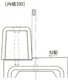
本体上部詳細図
